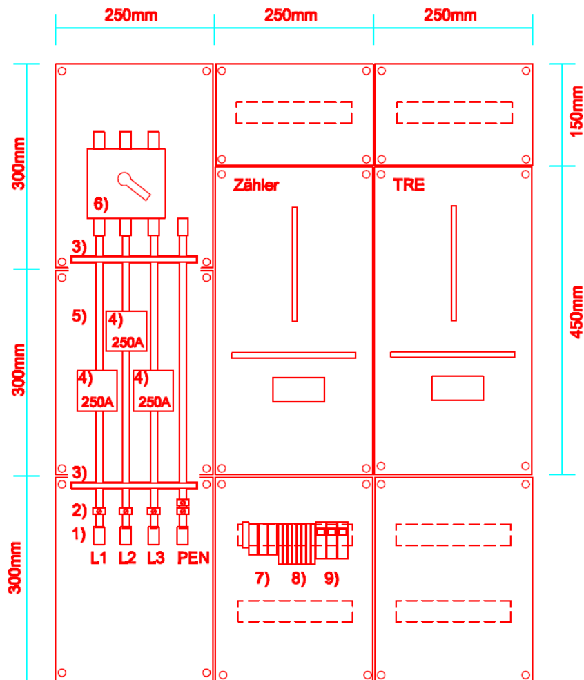
Bild: Wandlermessung - Einstöckiger Zählerschrank
