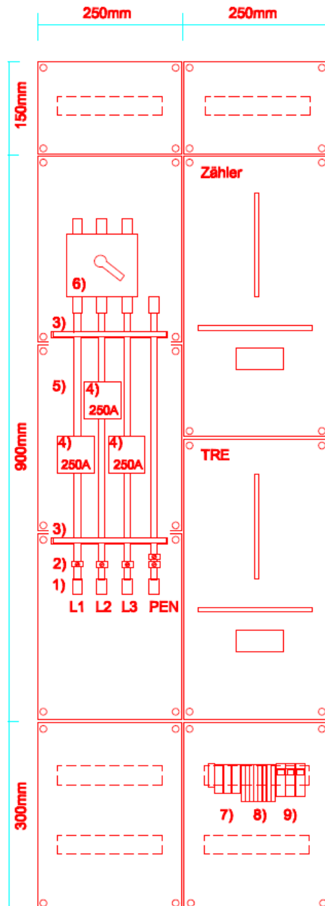
Bild: Wandlermessung - Doppelstöckiger Zählerschrank
