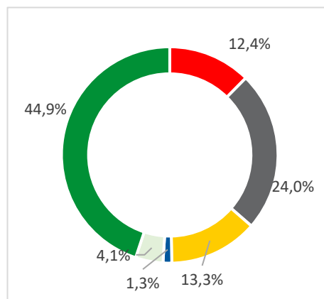
Stromerzeugung Deutschland
